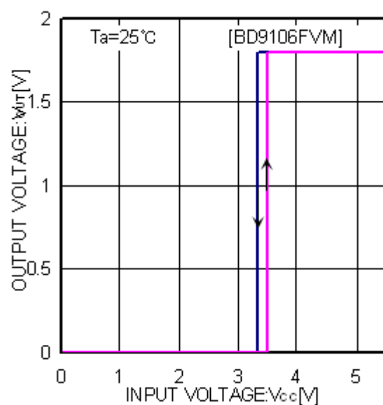
Fig.8 Vcc-Vout
