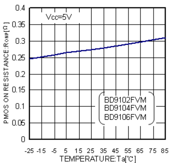
Fig.38 Ta-RONP
