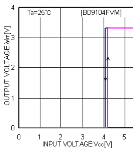
Fig.7 Vcc-Vout
