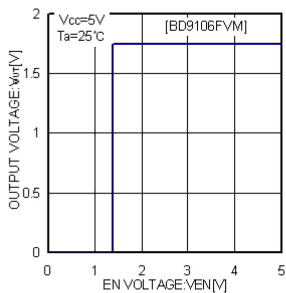
Fig.11 Ven-Vout
