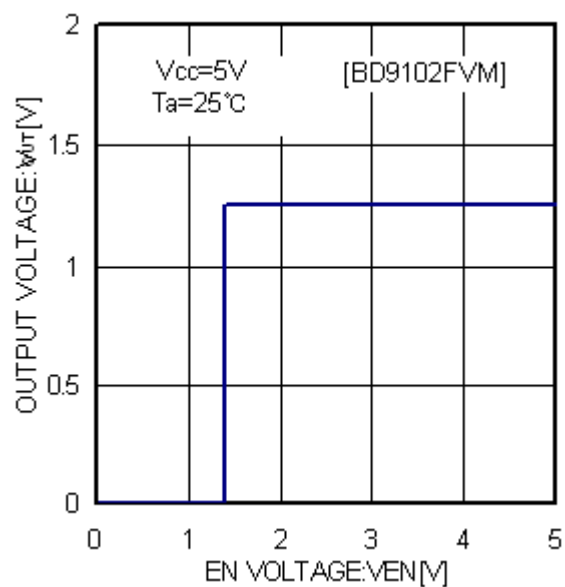
Fig.9 Ven-Vout
