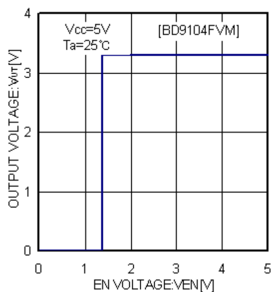
Fig.10 Ven-Vout
