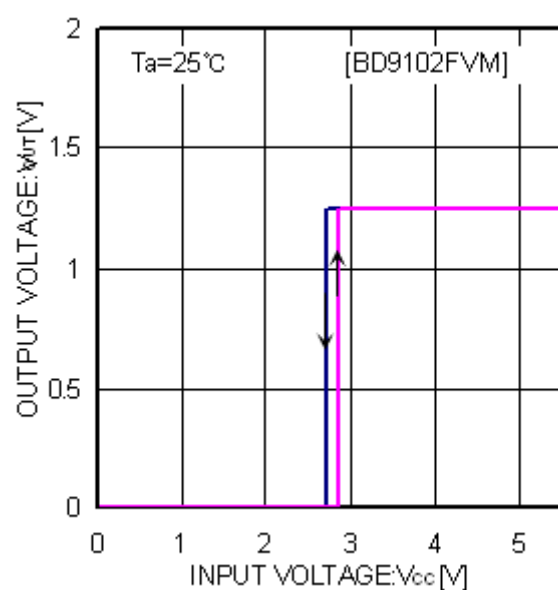
Fig.6 Vcc-Vout
