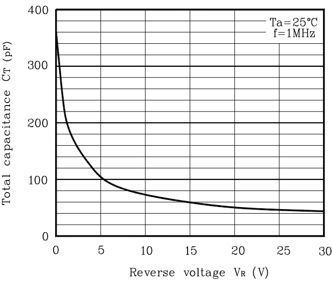
Fig. 3 C_T - V_R
