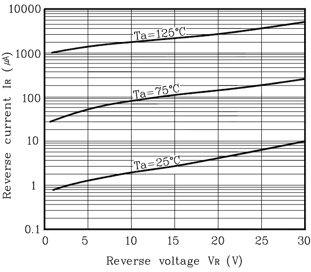
Fig. 2 I_R - V_R
