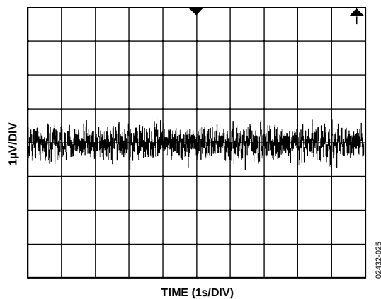
图 24. ADR421典型噪声电压0.1 Hz至10 Hz
