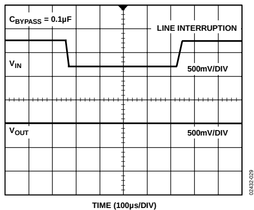
图 28. ADR421线性瞬态响应， C_{BYPASS} = 0.1\mu F
