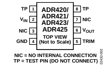
图 2. 8引脚SOIC或8引脚MSOP引脚配置
