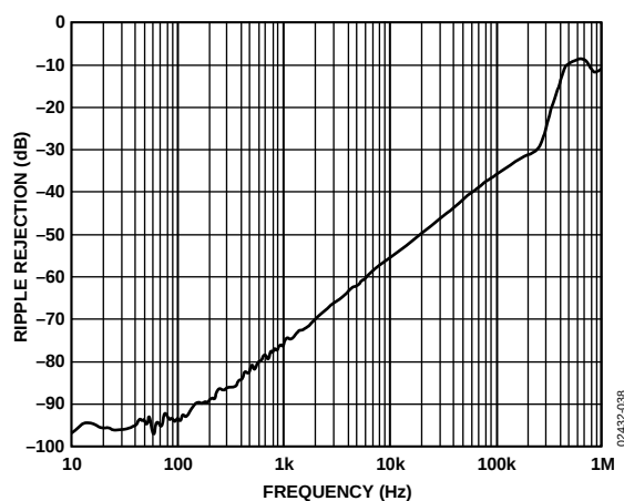
图 37. 纹波抑制与频率的关系
