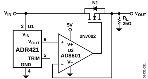
图 50. 精密升压输出调节器
