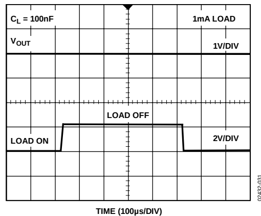
图 30. ADR421负载瞬态响应， C_L = 100\text{ nF}
