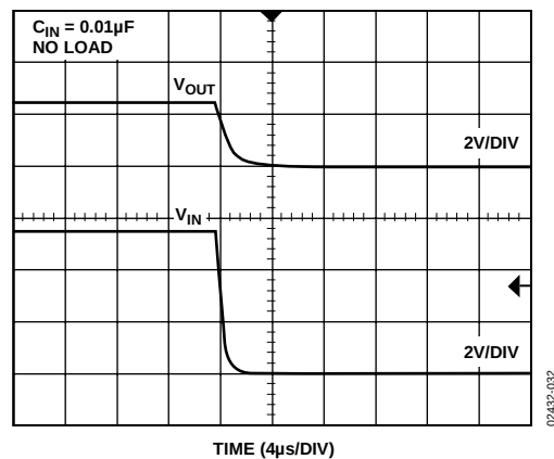
图 31. ADR421关闭响应
