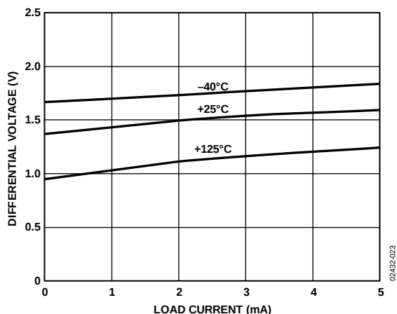
图 22. ADR425最小输入/输出差分电压与负载电流的关系
