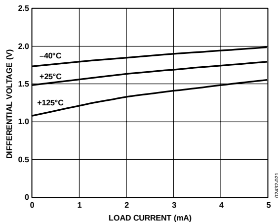
图 20. ADR421最小输入/输出差分电压与负载电流的关系
