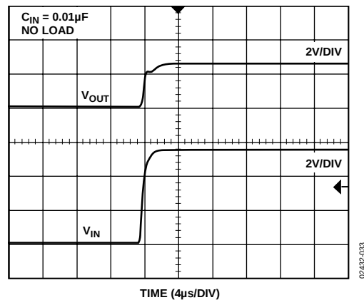
图 32. ADR421开启响应
