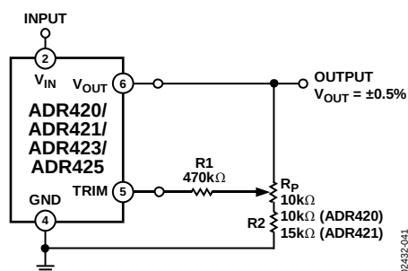
图 40. 输出调整功能
