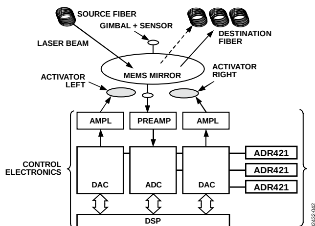
图 41. 全光路由器网络
