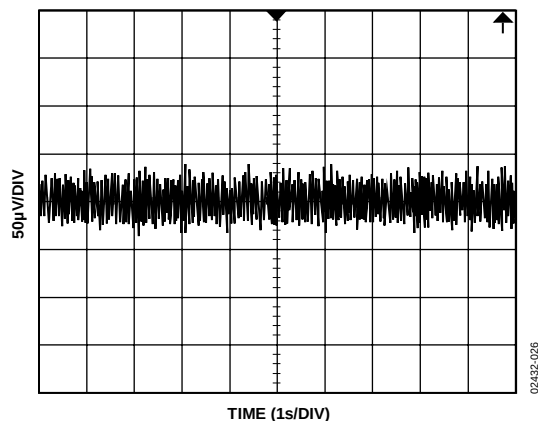
图 25. 典型噪声电压0 Hz至10 kHz
