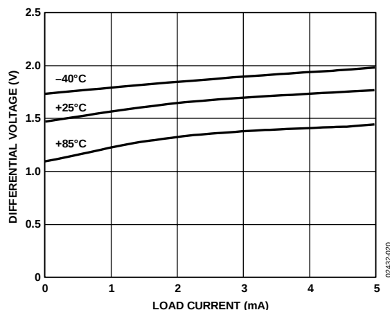
图 19. ADR420最小输入/输出差分电压与负载电流的关系
