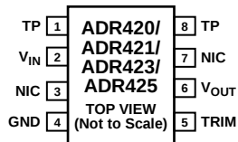
图 1. 8引脚SOIC或8引脚MSOP
