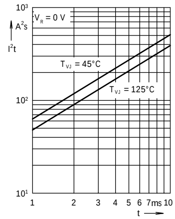
Fig. 5 I^2t versus time per diode
