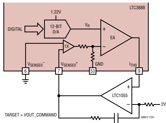
LTC3888/LTC3888-2
