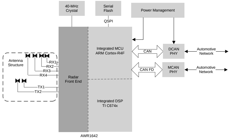
图 1-1. 适用于汽车 应用的自主雷达传感器
