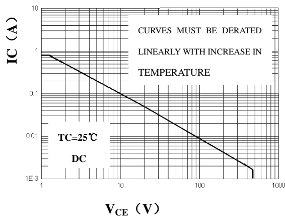
SOA
