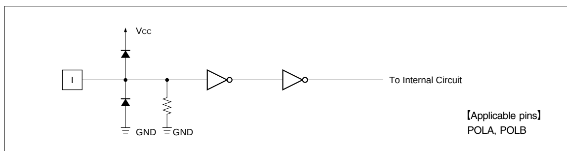
Fig. 2 Input Circuit (2)
