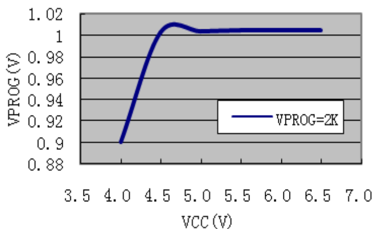
VPROG vs VCC
