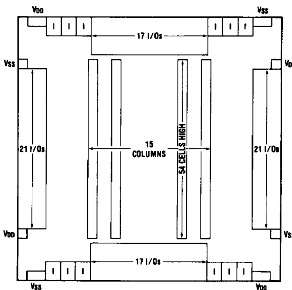
6225 Die Structure
