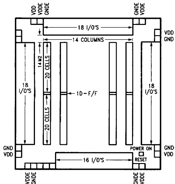
6218 Die Structure
