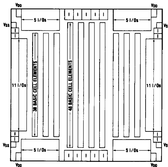
6212 Die Structure
