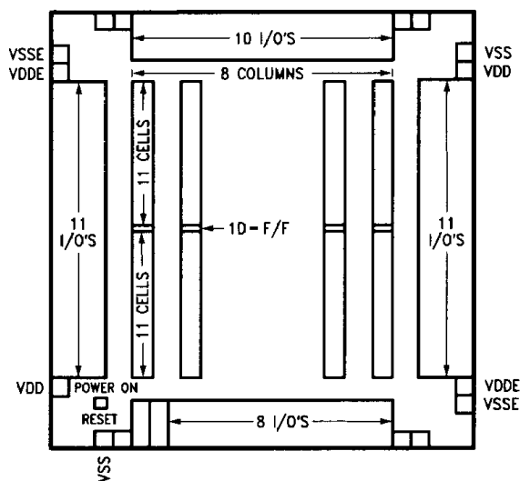
6206 Die Structure
