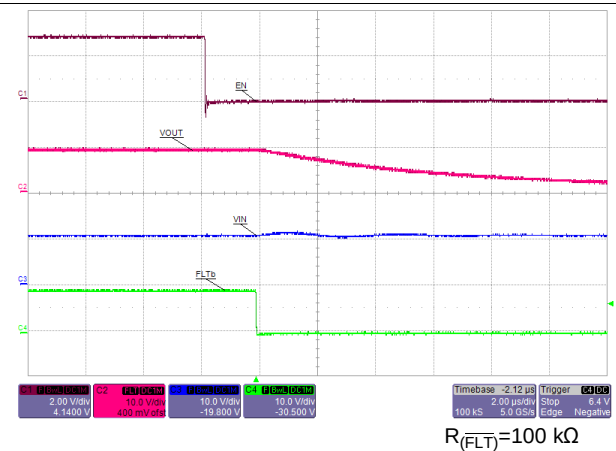
Figure 35. EN Turn OFF Delay : EN ↓ to Fault ↓
