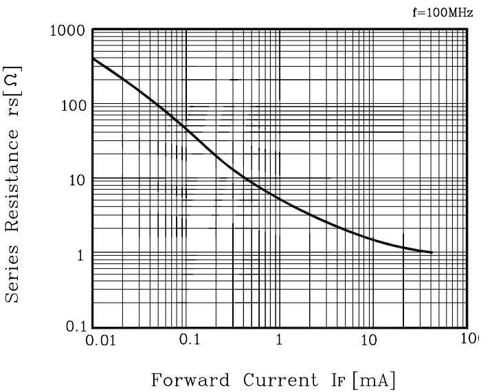
Fig. 2 r_s - I_F
