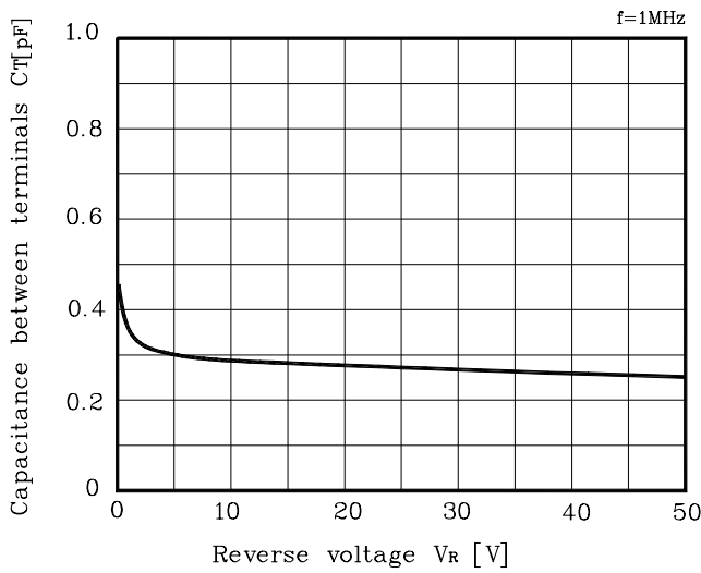
Fig. 1 C_T - V_R
