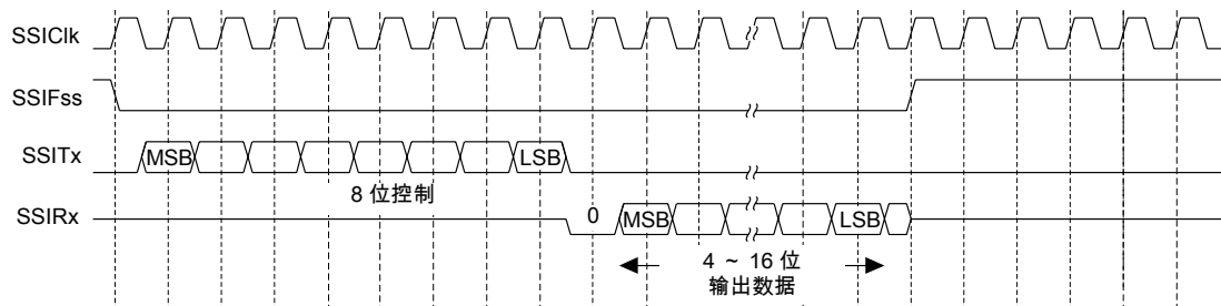
图 14-10. MICROWIRE 的帧格式 (单帧)
