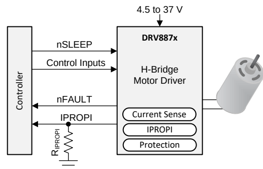
简化原理图
