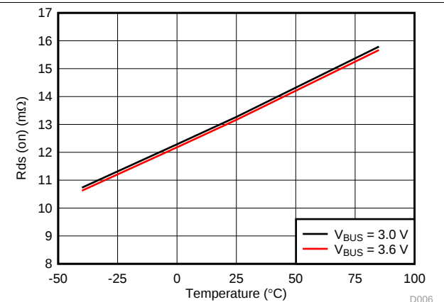
图 6. R_{ds(on)} vs Temperature
