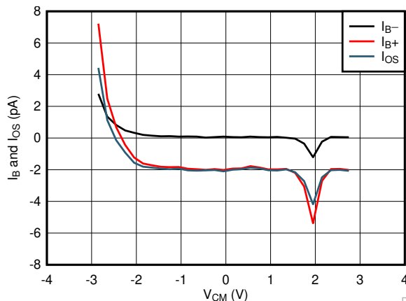
图 7-7. I_B 和 I_{OS} 与共模电压间的关系
