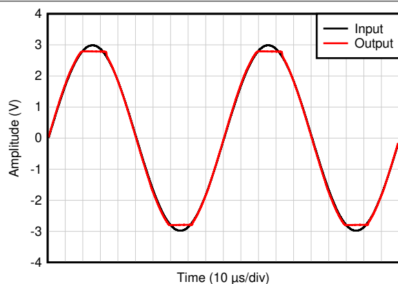
图 7-59. 无相位反转
