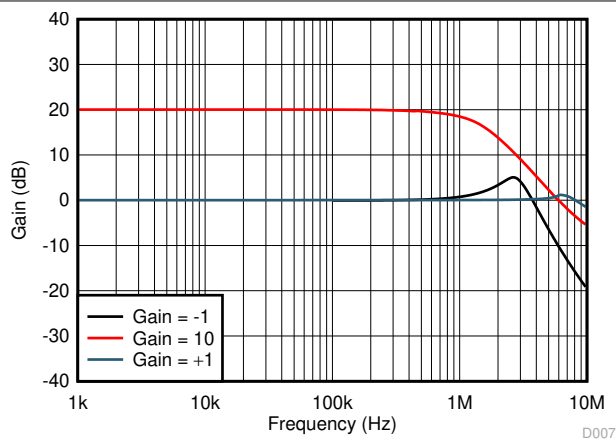
图 7-10. 闭环增益与频率间的关系
