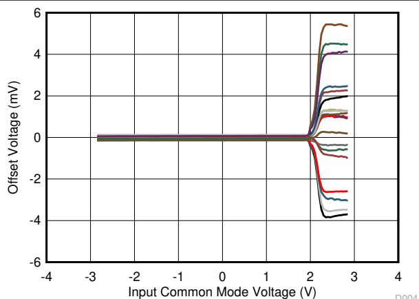
图 7-4. 失调电压与共模电压间的关系
