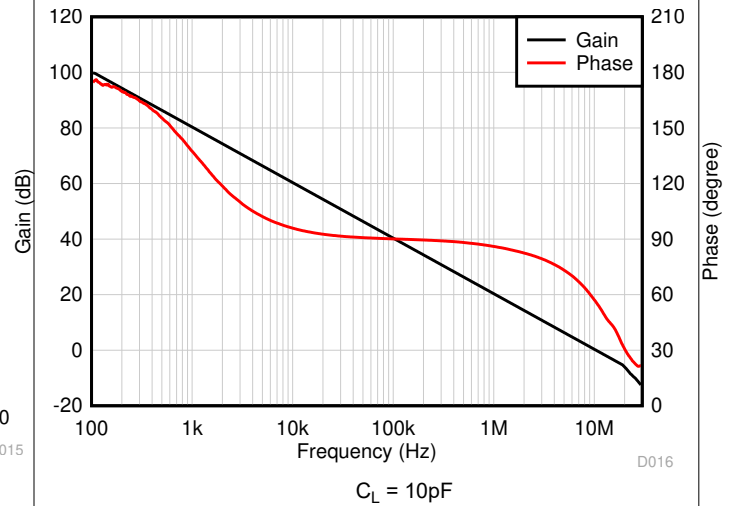
图 7-54. 开环增益和相位与频率间的关系
