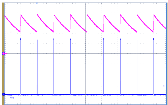
Time Scale: 100 μs/Div CH1: V_{SW} , 4 V/Div CH4: I_L , 200 mA/Div
