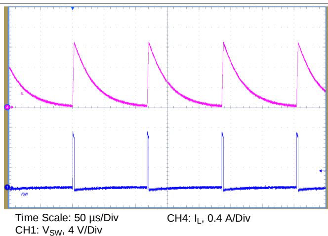
图 83. Short Circuit
