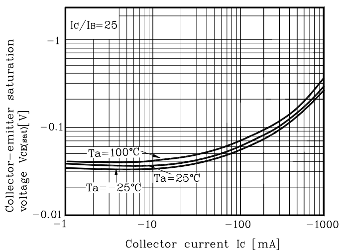
Fig. 5 V_{CE(SAT)} - I_c
