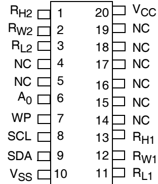
20 Pin TSSOP
