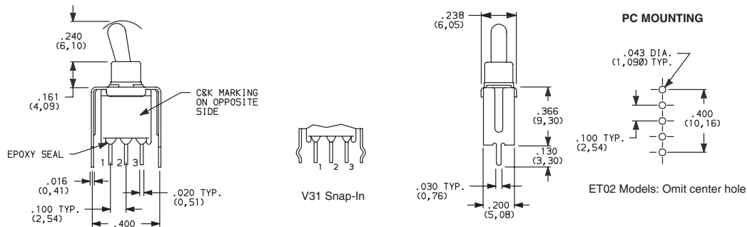
ET01MD1V3BE SPDT
