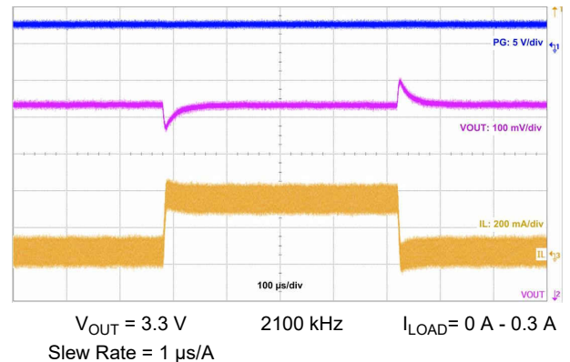
图 9-32. Load Transient
