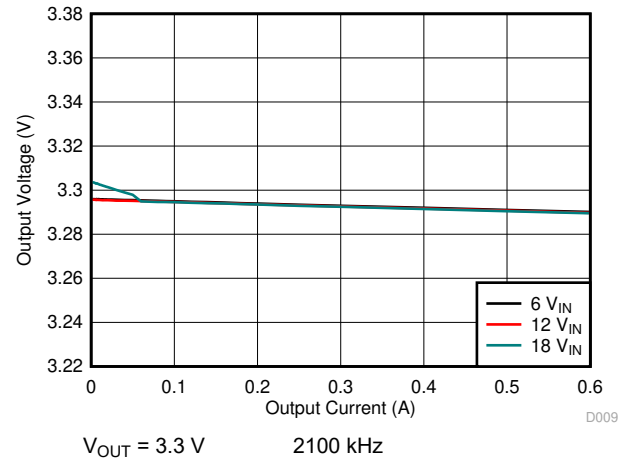
图 9-28. Load Regulation
