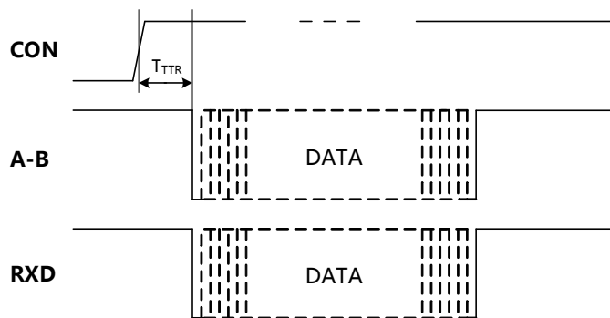
图 2. TDM(3)485CT模块数据接收时序图
