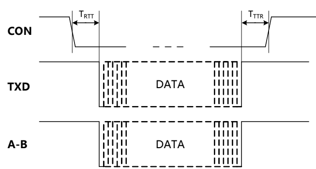
图 1. TDM(3)485CT模块数据发送时序图
