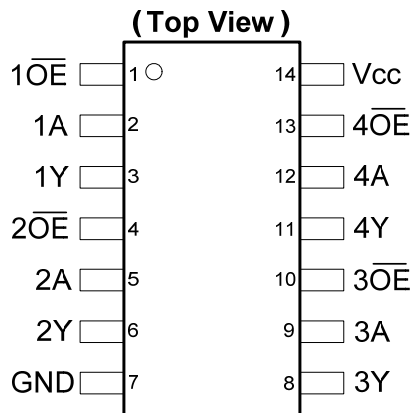
SO-14 / TSSOP-14
