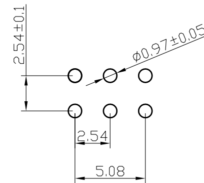
PCB开孔
