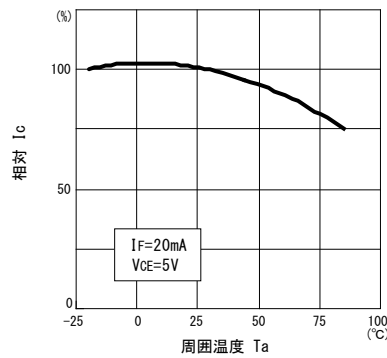
■ 相対光電流/周囲温度特性 相対 I_C/T_a
