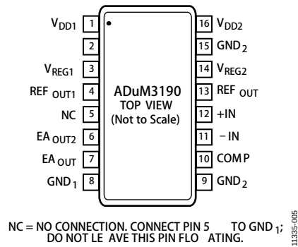
图3. 引脚配置
