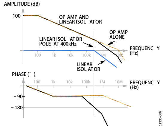
图21. 波特图1
