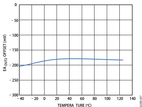
图14. EA OUT2 失调与温度的关系
