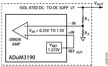
图25. 设置输出电压
