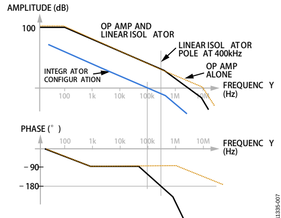
图22. 波特图2
