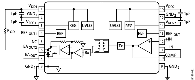
图20. 测试电路3
