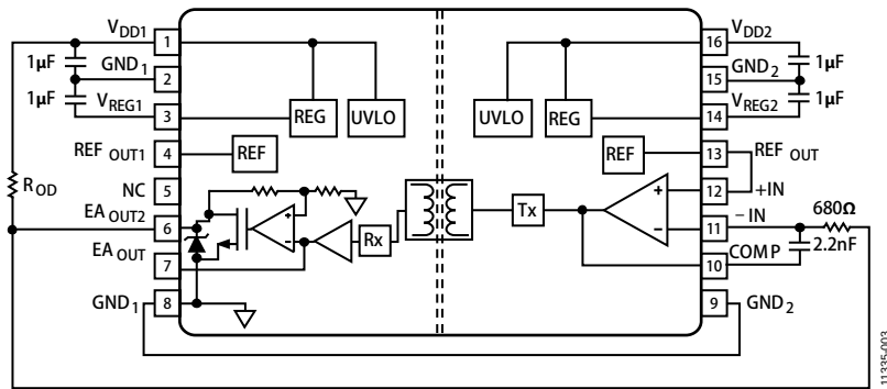
图19. 测试电路2
