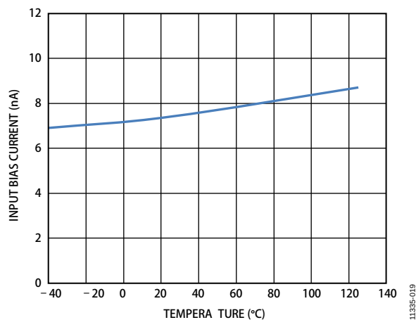
图6. 输入偏置电流+IN、-IN与温度的关系
