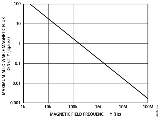
图27. 最大允许外部磁通密度
