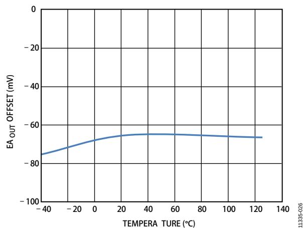
图13. EA OUT 失调与温度的关系
