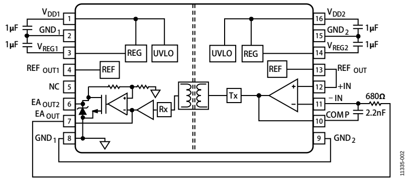
图18. 测试电路1
