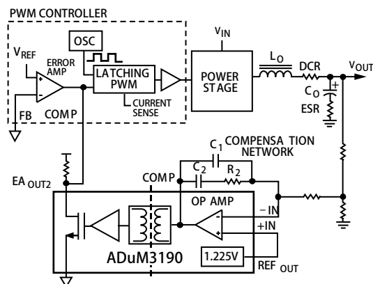
图23. 应用功能框图1
