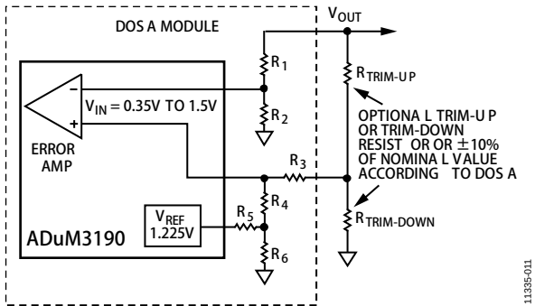
图26. DOSA模块
