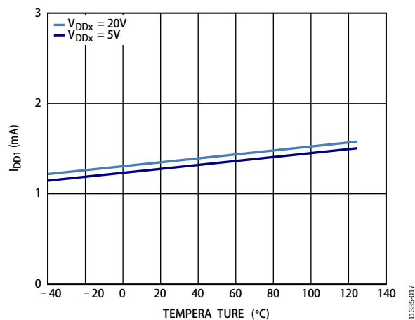
图4. 典型 I_{DD1} 电源电流与温度的关系
