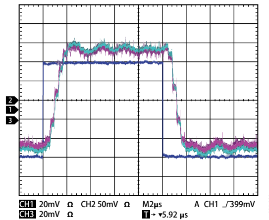
图17. 输出方波响应; 测试电路3, 通道1 = +IN, 通道2 = EA_{OUT} , 通道3 = EA_{OUT2}
