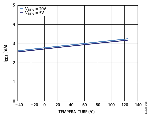
图5. 典型 I_{DD2} 电源电流与温度的关系
