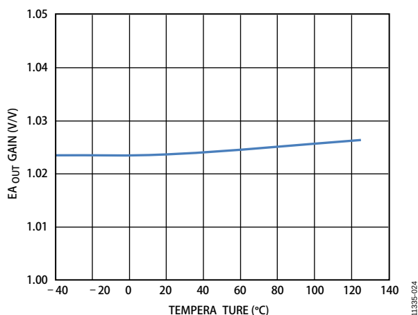
图11. EA OUT 增益与温度的关系
