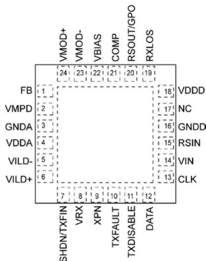
24-Pin QFN
