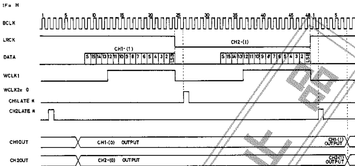
タイミングチャート(1)
