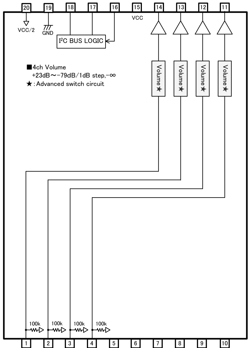
Fig.19 BD3464FV
