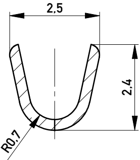
Schnitt B-B M 10:1
