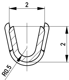
Schnitt A-A M 10:1
