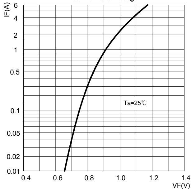
图3: 正向电压曲线 FIG3: Forward Voltage
