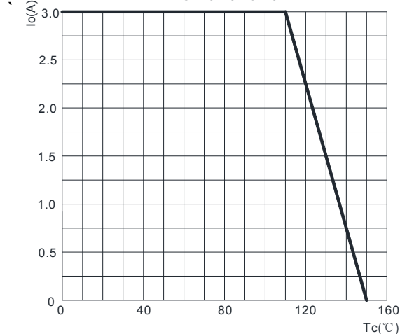
图1: I o -T c 曲线 FIG1:I o -T c Curve
