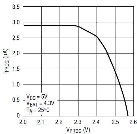
PROG 引脚上拉电流 vs PROG 引脚电压 (上拉电流)
