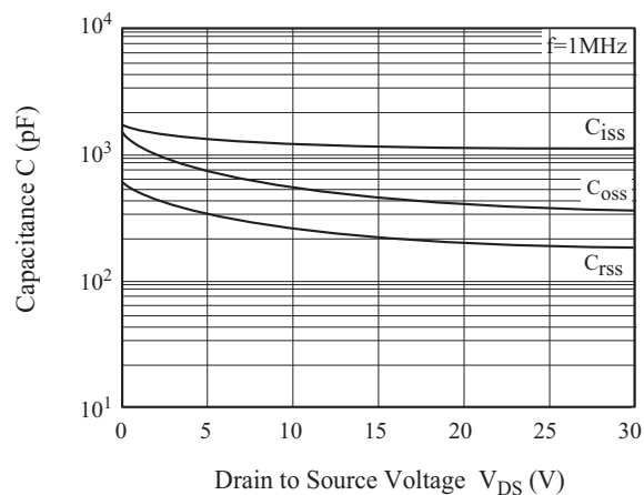
Fig8. C - V_{DS}
