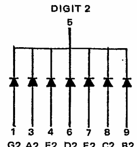
CS-323 COMMON CATHODE
