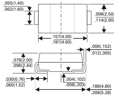
SMA/DO-214AC
