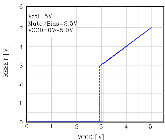
Fig. 6 V_{CCD} - RESET
