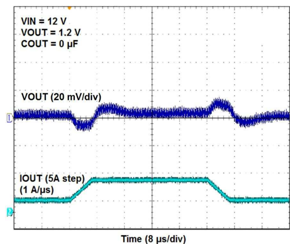
瞬态响应
