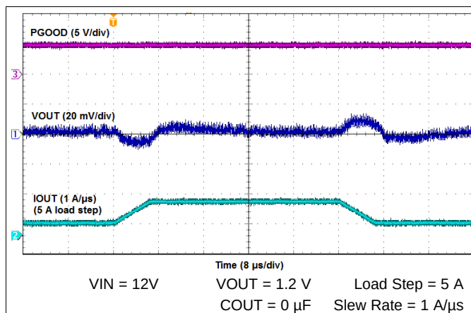
图 12. Transient Response
