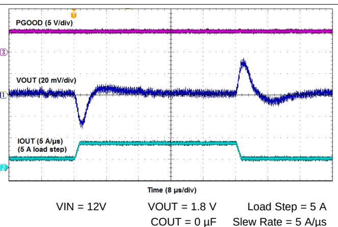
图 15. Transient Response
