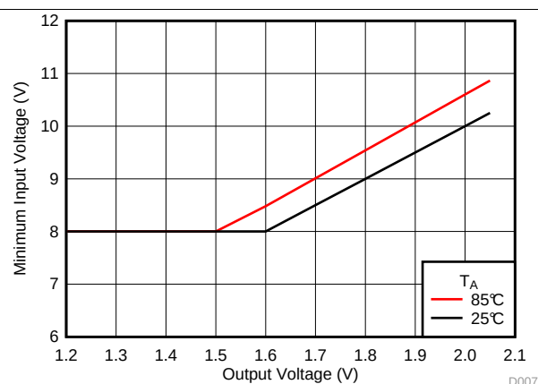
图 11. Minimum Input Voltage
