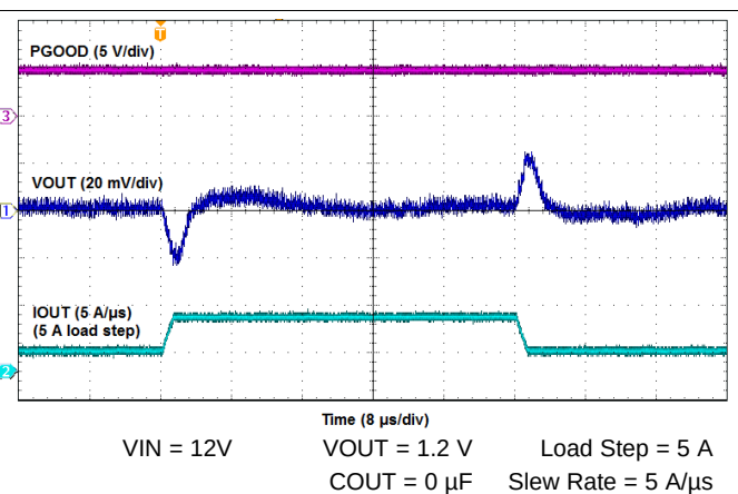
图 13. Transient Response
