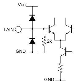
24pin (27pin)
