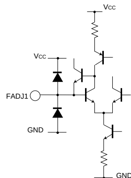
3pin (43pin)
