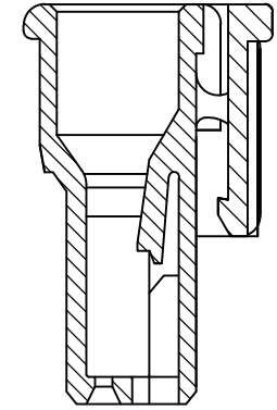
SECT A-A
