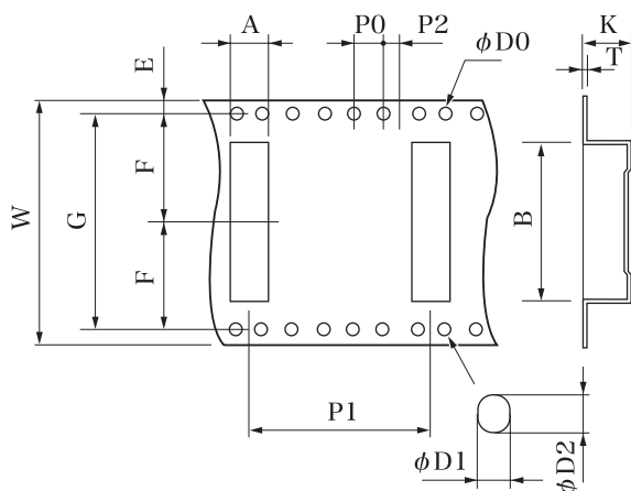
10 □ -1A TYPE
