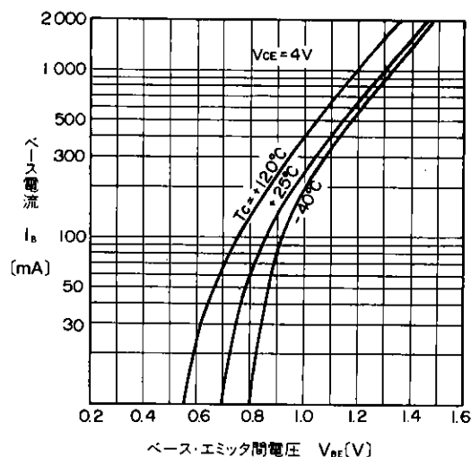
入力特性 Input Characteristics
