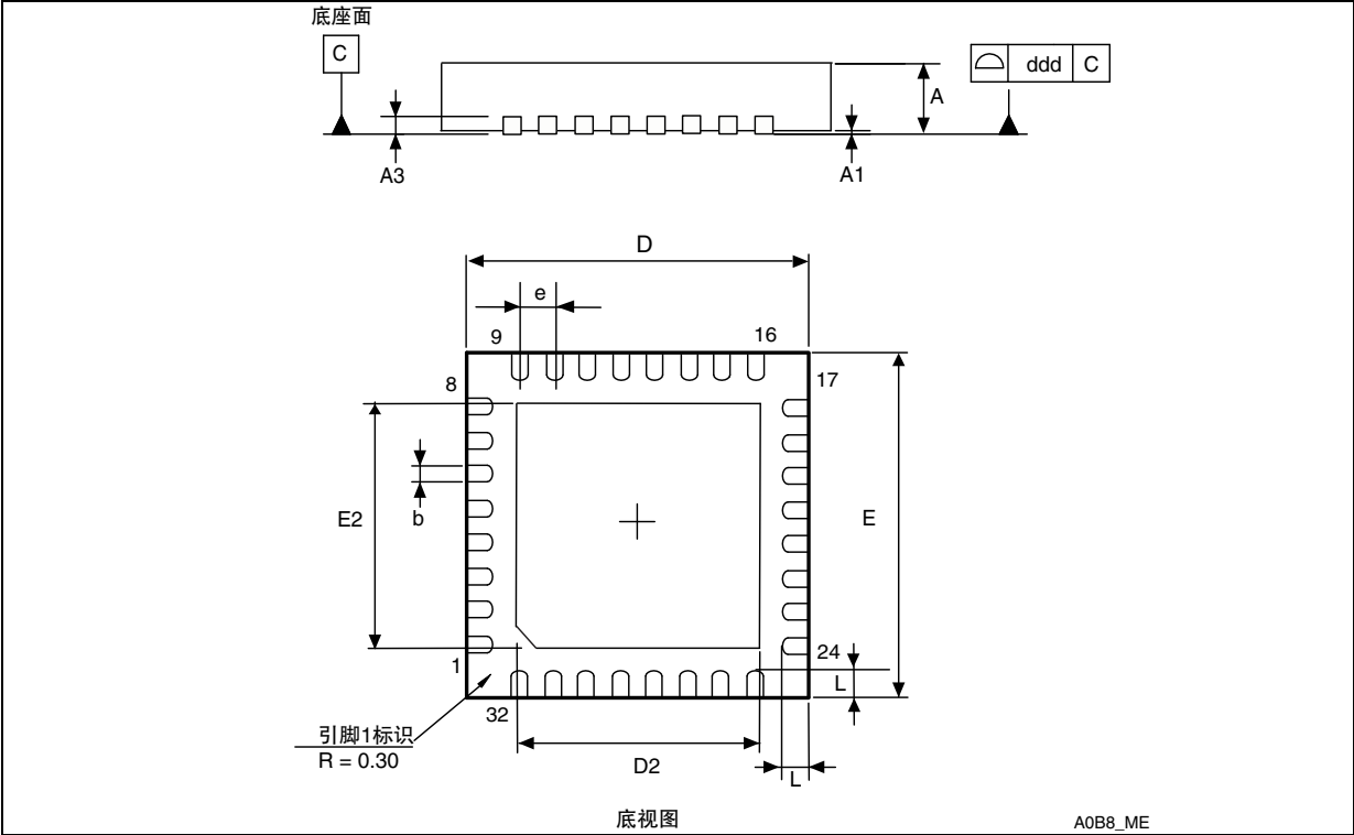
图 35. UFQFPN32 - 5 × 5 mm， 32 引线，超薄紧密排列正方扁平无引线封装图
