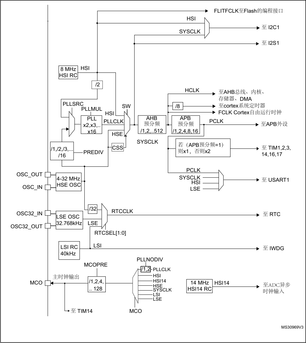
图 2. 时钟树
