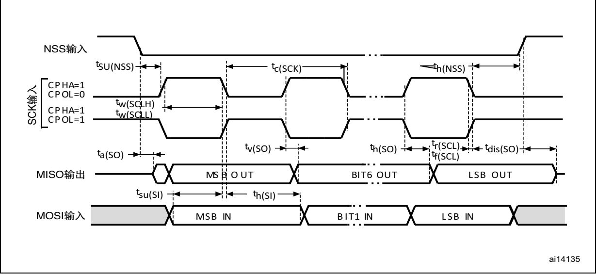
图 26. SPI 时序图 – 从模式且 CPHA = 1
