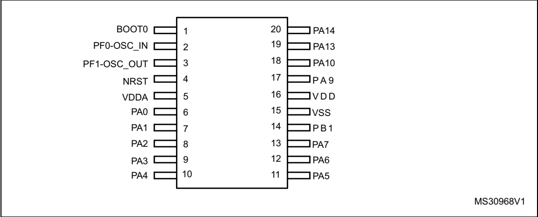
图 7. TSSOP20 20 引脚封装引脚排列
