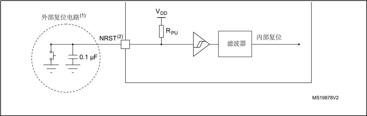
图 22. 推荐的 NRST 引脚保护
