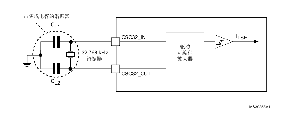
图 16. 采用 32.768 kHz 晶振的典型应用
