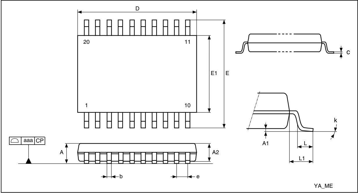
图 39. TSSOP20 - 20 引脚纤薄紧缩小尺寸
