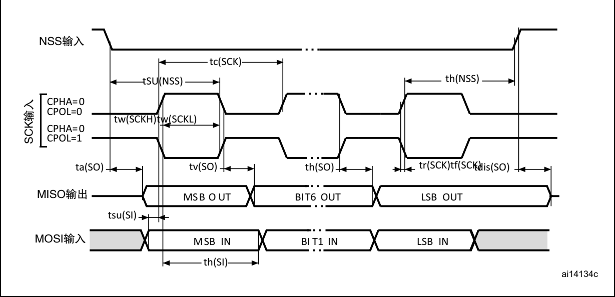
图 25. SPI 时序图 – 从模式且 CPHA = 0
