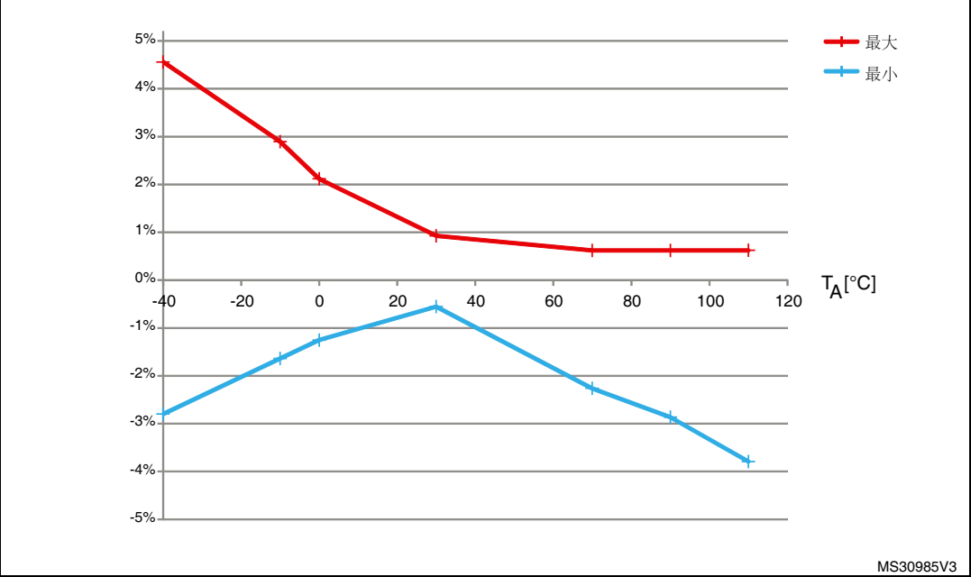
图 17. HSI 振荡器精度特性结果
