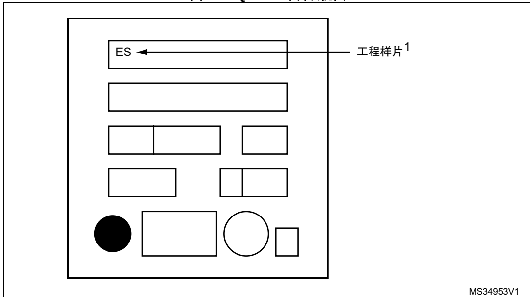
图 34. LQFP32 封装顶视图
