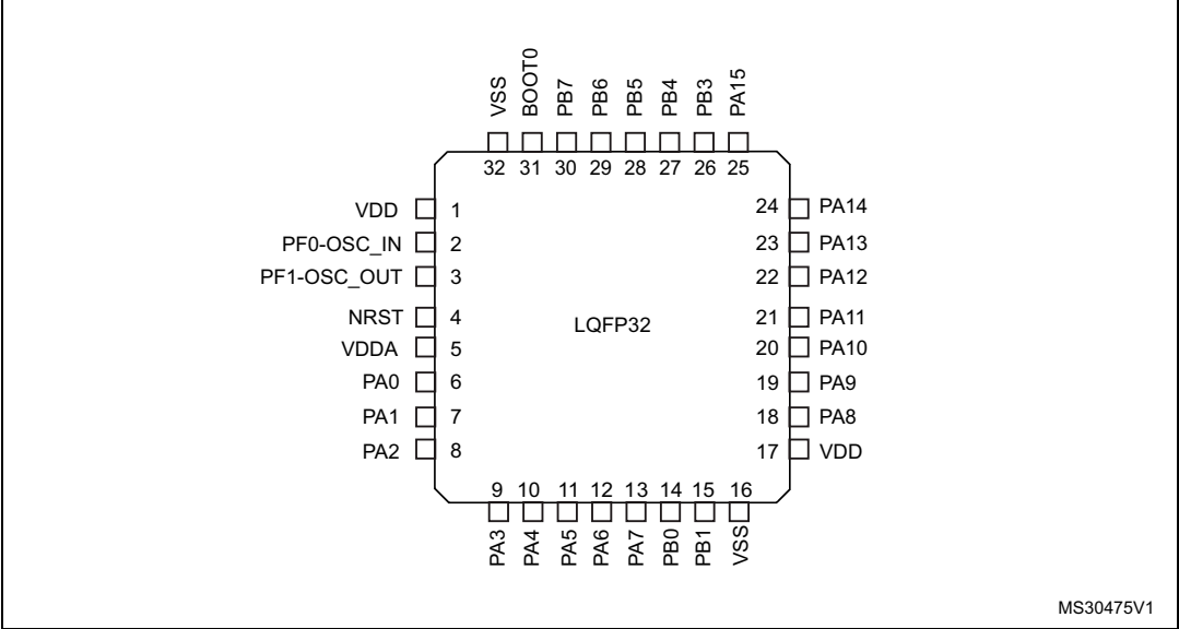
图 4. LQFP32 32 引脚封装引脚排列
