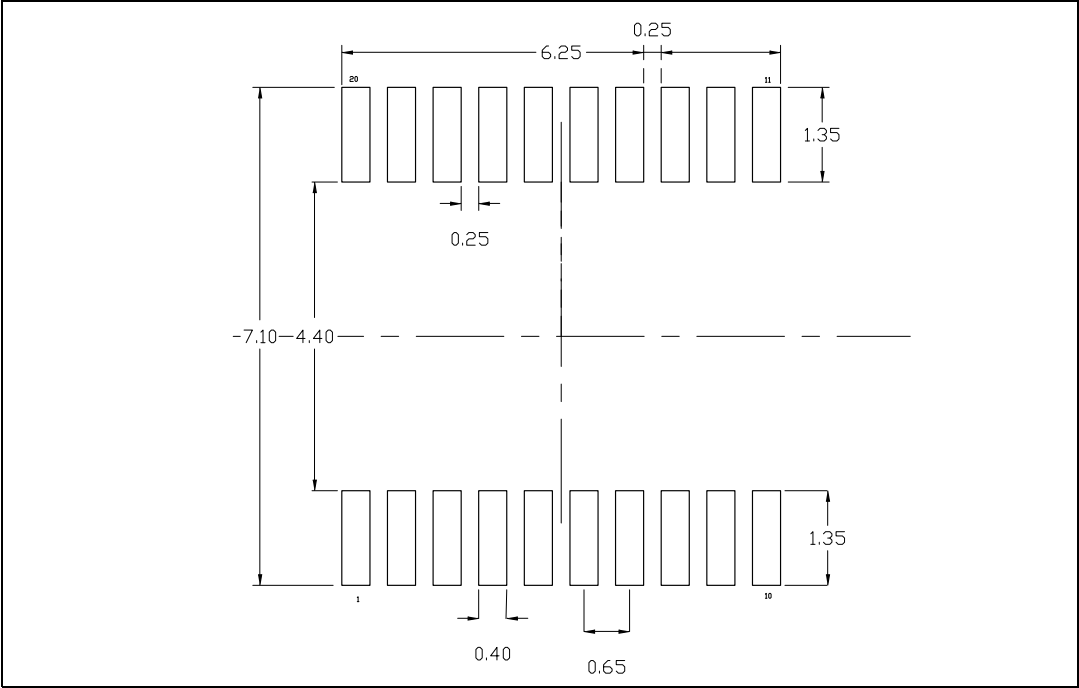
图 40. TSSOP20 建议尺寸
