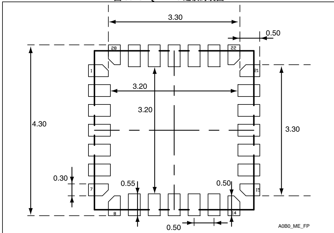
图 38. UFQFPN28 建议封装图
