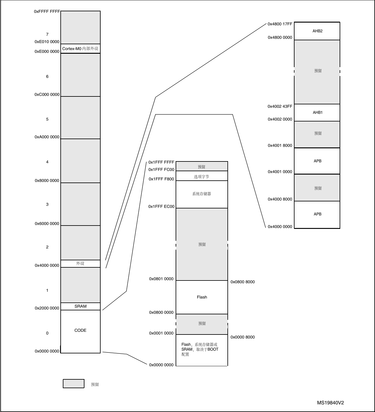
图 8. STM32F031x4/x6 存储器映射
