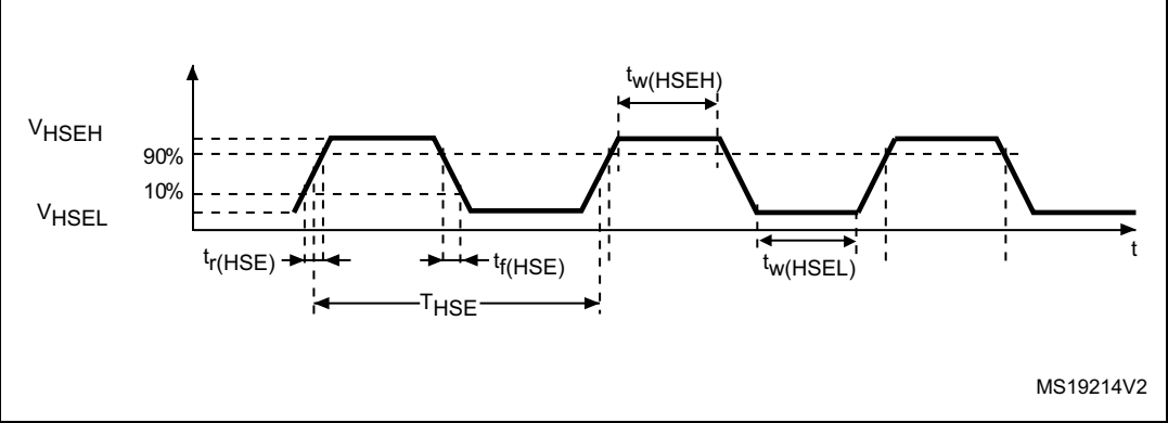
图 13. 高速外部时钟源的交流时序图
