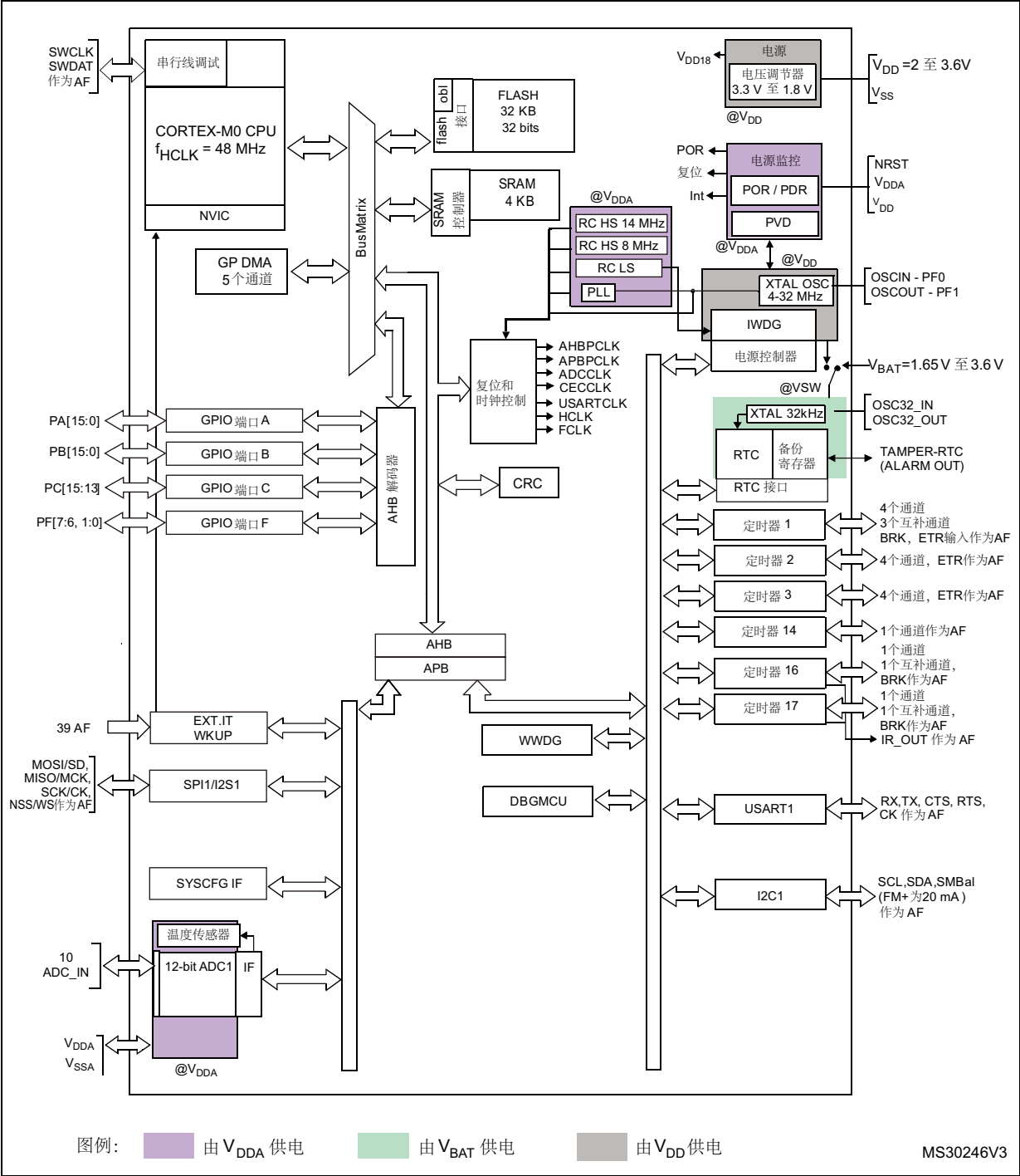
图 1. 框图
