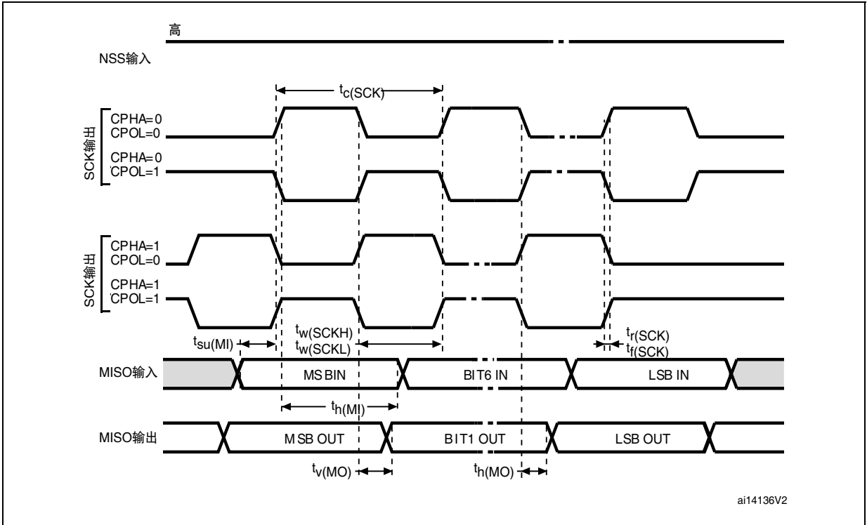
图 27. SPI 时序图 – 主模式
