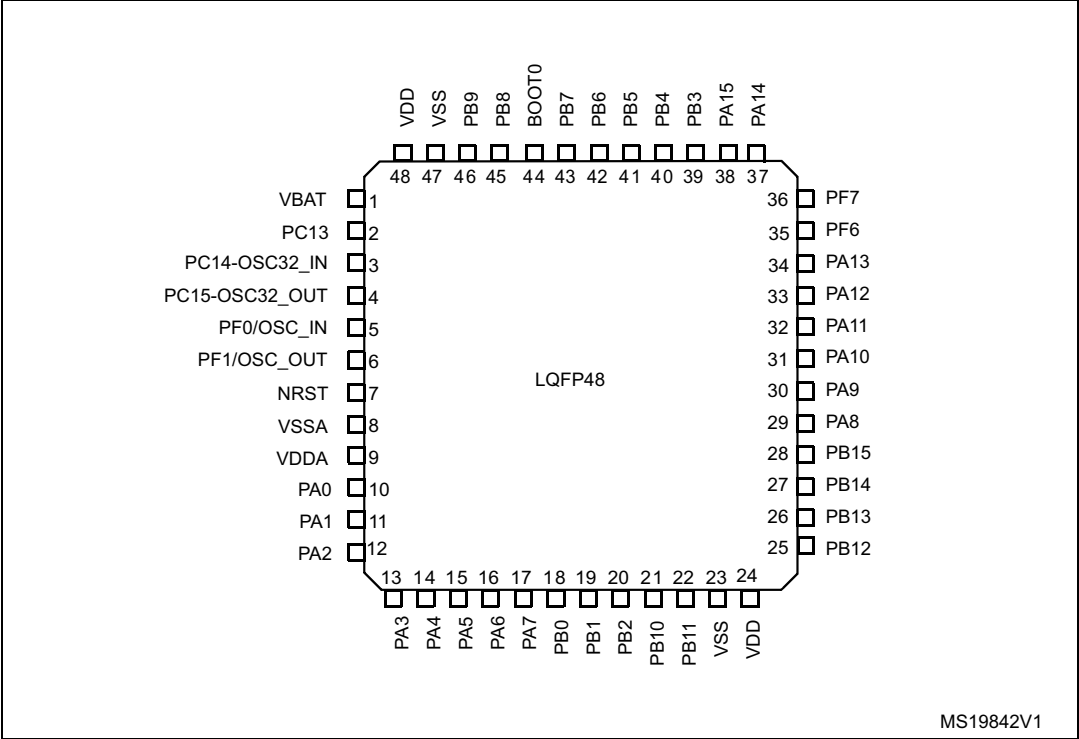
图 3. LQFP48 48 引脚封装引脚排列
