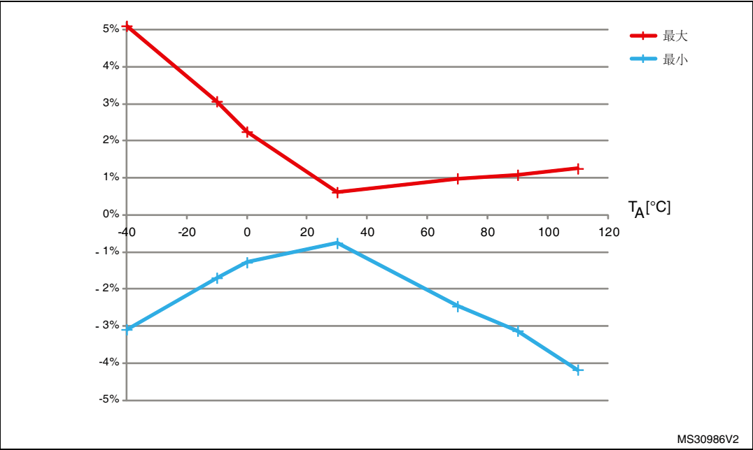
图 18. HSI14 振荡器精度特性结果
