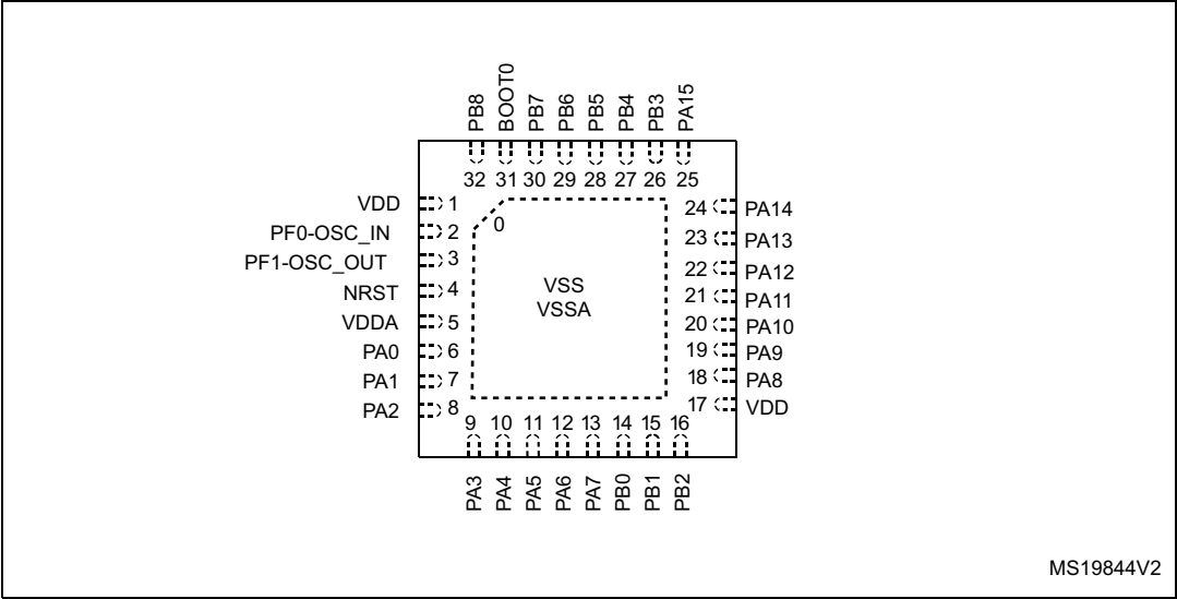
图 5. UFQFPN32 32 引脚封装引脚排列
