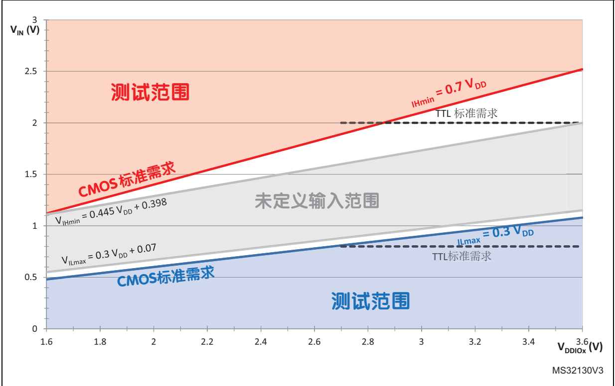
图 19. TC 和 TTa I/O 输入特性
