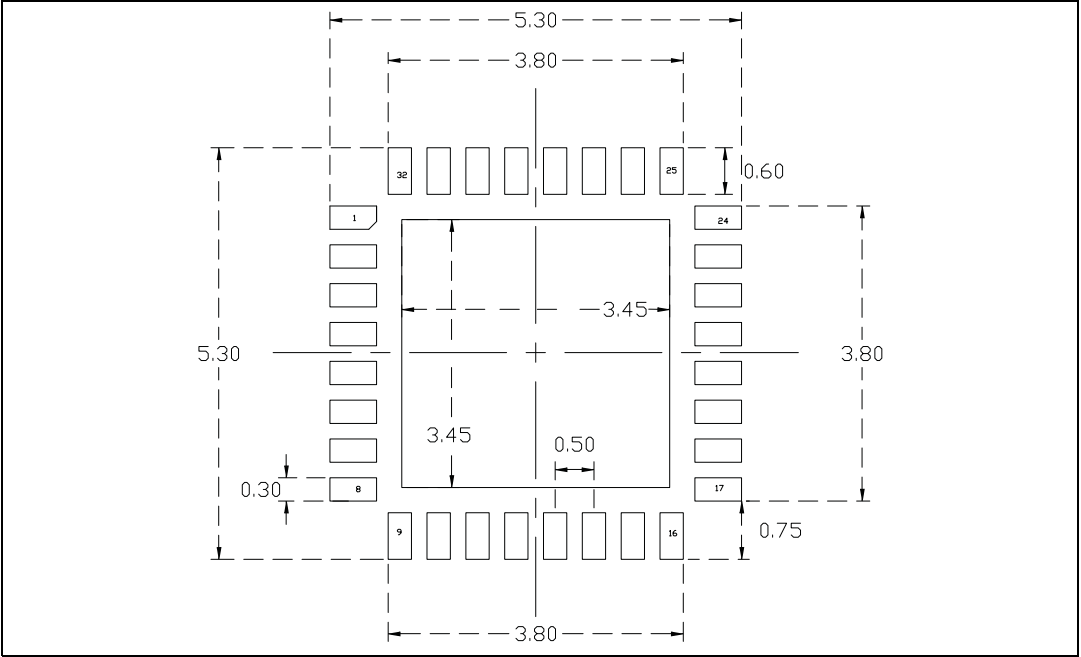
图 36. UFQFPN32 建议封装图
