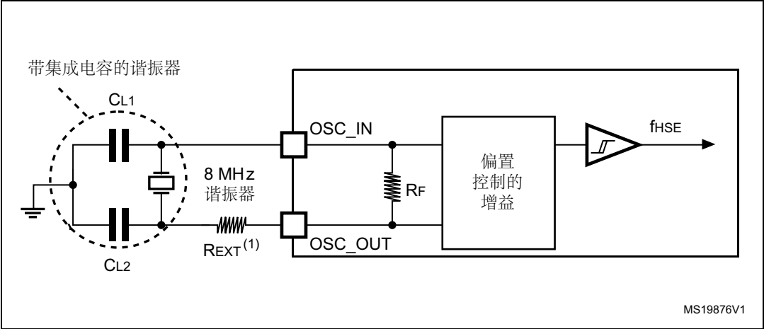
图 15. 采用 8 MHz 晶振的典型应用
