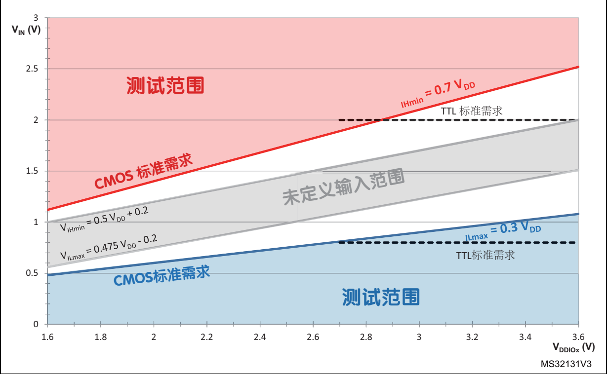
图 20. 5 V 容限（FT 和 FTf） I/O 输入特性
