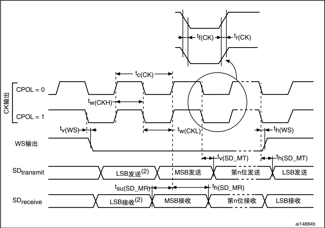
图 29. I2S 主模式时序图（Philips 协议）
