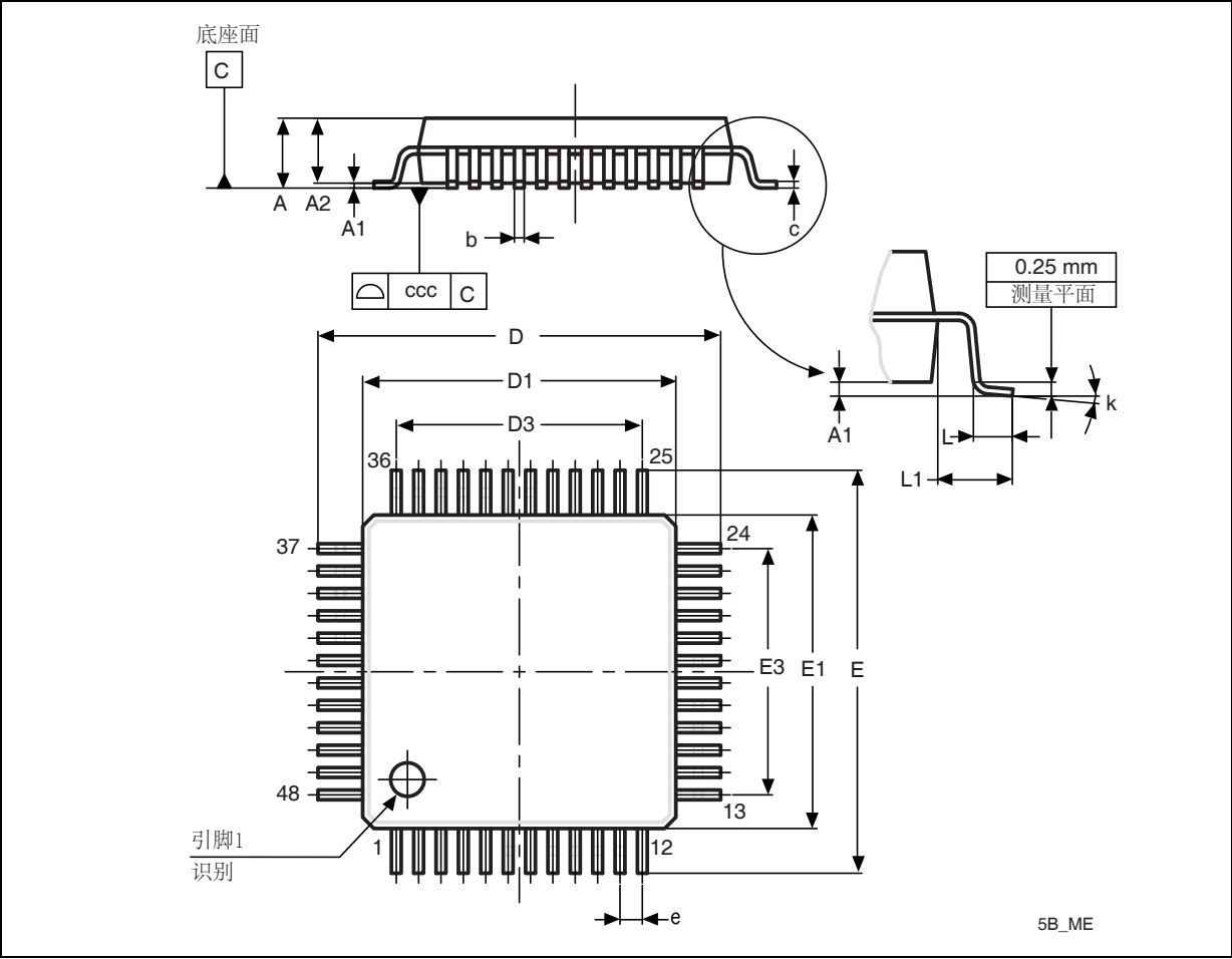
图 30. LQFP48 – 7 × 7 mm 48 引脚薄型正方扁平封装图
