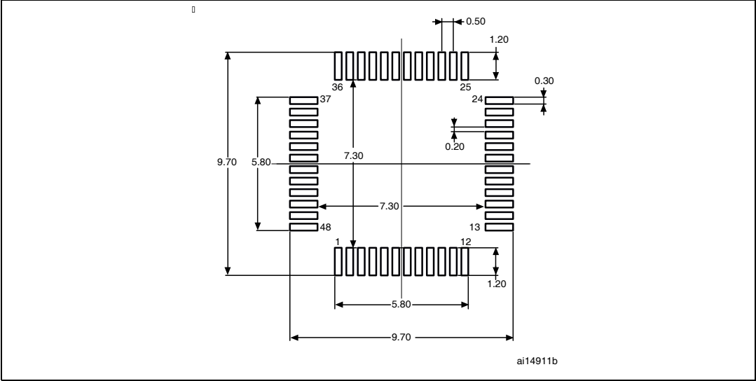
图 31. LQFP48 建议封装图
