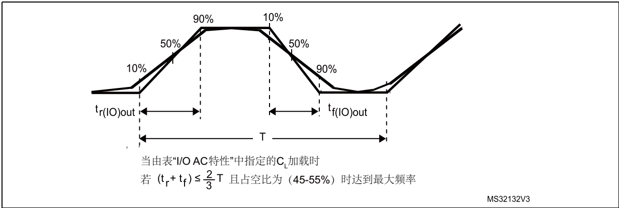
图 21. I/O 交流特性定义
