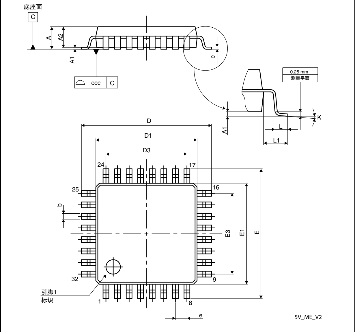
图 32. LQFP32 – 7 × 7 mm 32 引脚薄型正方扁平封装图
