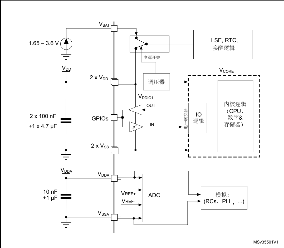
图 11. 电源方案
