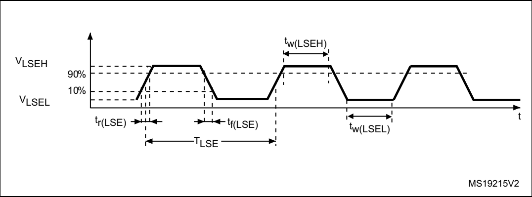
图 14. 低速外部时钟源的交流时序图
