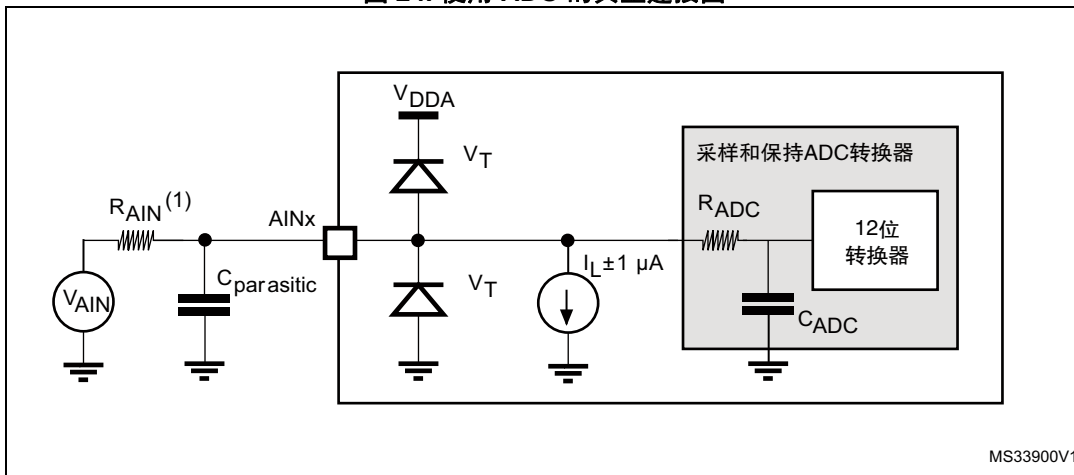
图 24. 使用 ADC 的典型连接图
