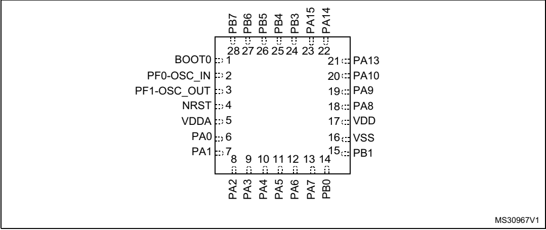
图 6. UFQFPN28 28 引脚封装引脚排列
