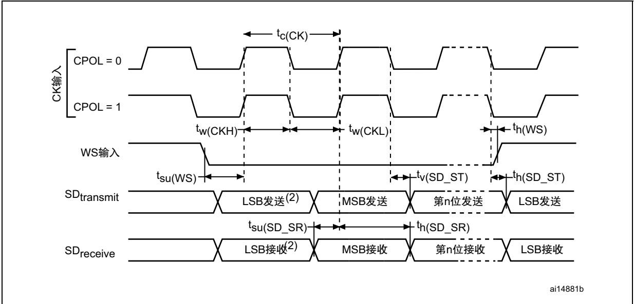
图 28. I2S 从模式时序图（Philips 协议）
