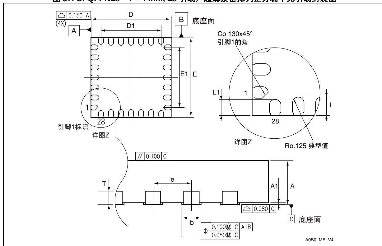
图 37. UFQFPN28 - 4 × 4 mm, 28 引线, 超薄紧密排列正方扁平无引线封装图
