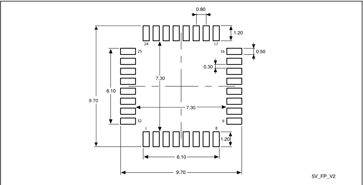
图 33. LQFP32 建议封装图
