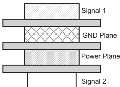
图 45. Example Layout
