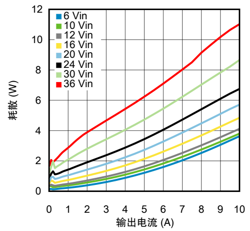
输出 1.0V，环境温度为 25℃ 时的耗散
