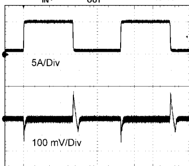
瞬态响应 12 V IN , 1.2 V OUT 1 至 10A 阶跃
