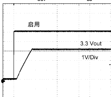
3.3 V OUT 软启动, 无 C SS
