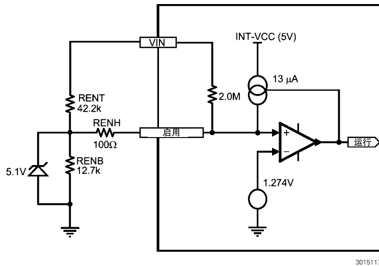
图 1：启用输入细节
