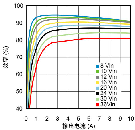
输出 5.0V，环境温度为 85℃ 时的效率
