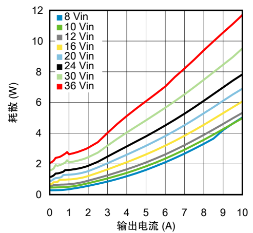
输出 5.0V，环境温度为 85℃ 时的耗散
