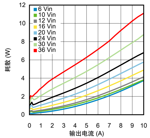
输出 1.2V，环境温度为 25℃ 时的耗散
