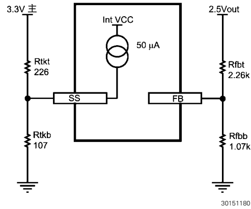
图 2: 跟踪选择输入详图
