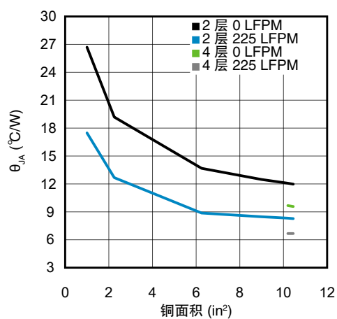
\theta_{JA} 与铜散热面积的关系
