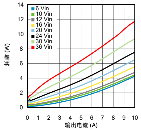
输出 1.2V, 环境温度为 85°C 时的耗散
