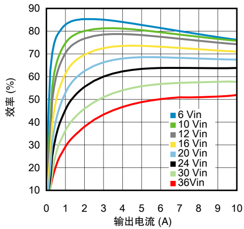
输出 1.2V，环境温度为 25℃ 时的效率
