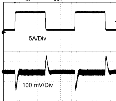
瞬态响应 12 V IN , 5.0 V OUT 1 至 10A 阶跃
