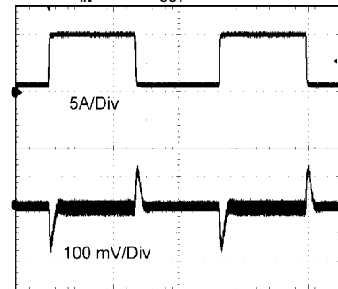
瞬态响应 12 V IN , 3.3 V OUT 1 至 10A 阶跃
