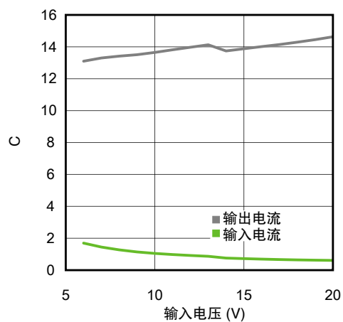
短路电流与输入电压的关系
