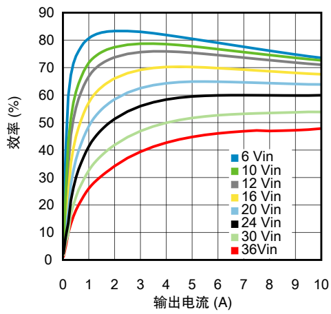
输出 1.0V，环境温度为 25℃ 时的效率
