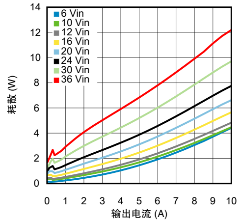
输出 1.5V, 环境温度为 85°C 时的耗散
