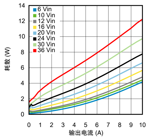
输出 1.0V, 环境温度为 85°C 时的耗散
