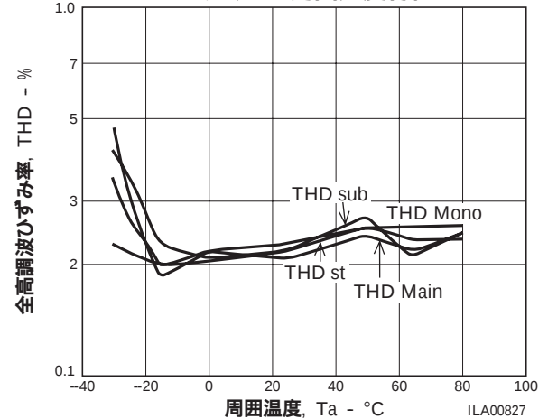
ひずみ -- 周囲温度特性
