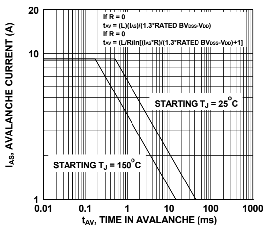
图 12. 非箝位感性开关特性
