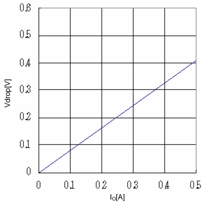
Fig.22 Minimum dropout Voltage 2 ( V_{cc}=4.5 V、 T_a=25 °C)
