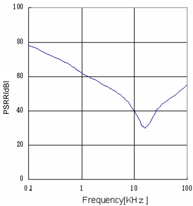
Fig.21 PSRR ( I_o=0 mA)
