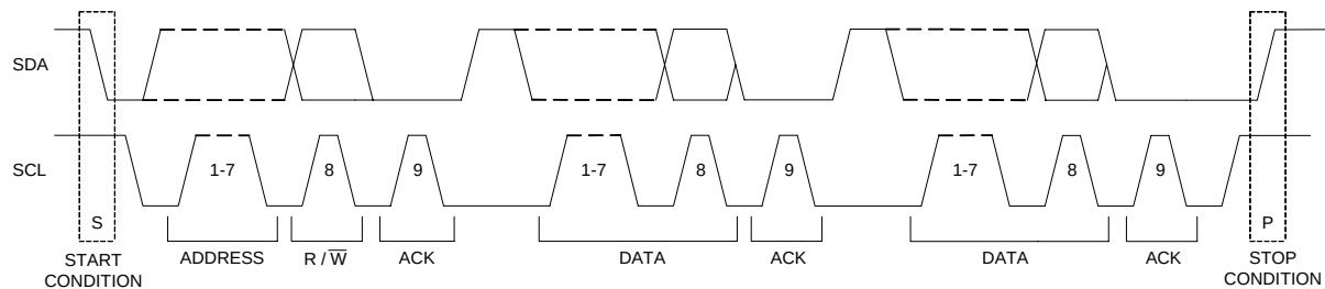
Fig.4 I²C format
