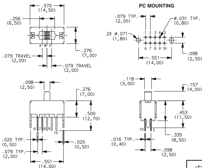
OS203011MV9QS1 DP3T
