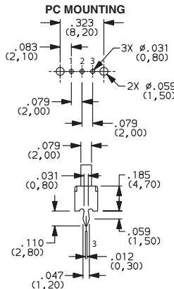
OS102011MS2QN1 SPDT
