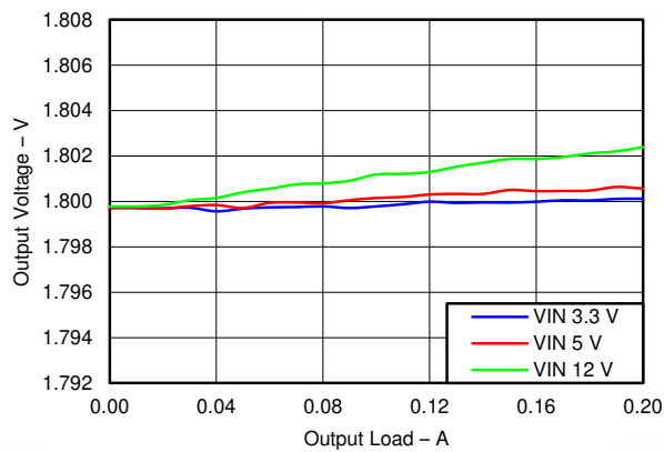
图 6-9. LDO1, Load Regulation
