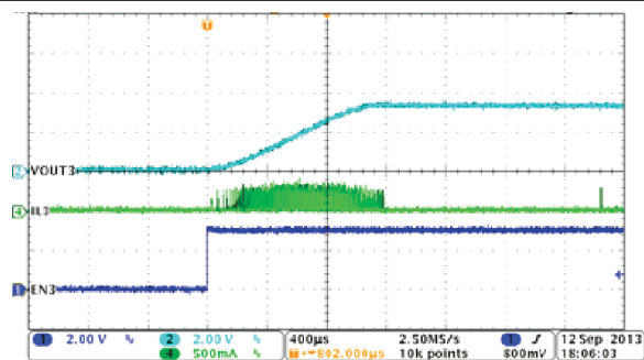
图 8-7. Buck3, Soft-Start With No Load
