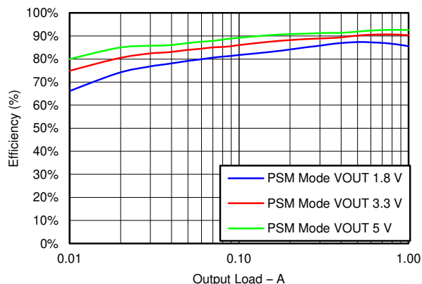
图 6-2. Buck2 Efficiency
