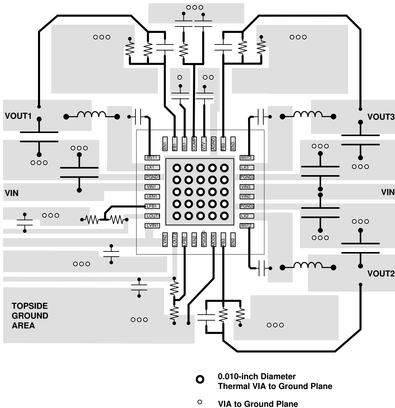
图 8-35. PCB Layout
